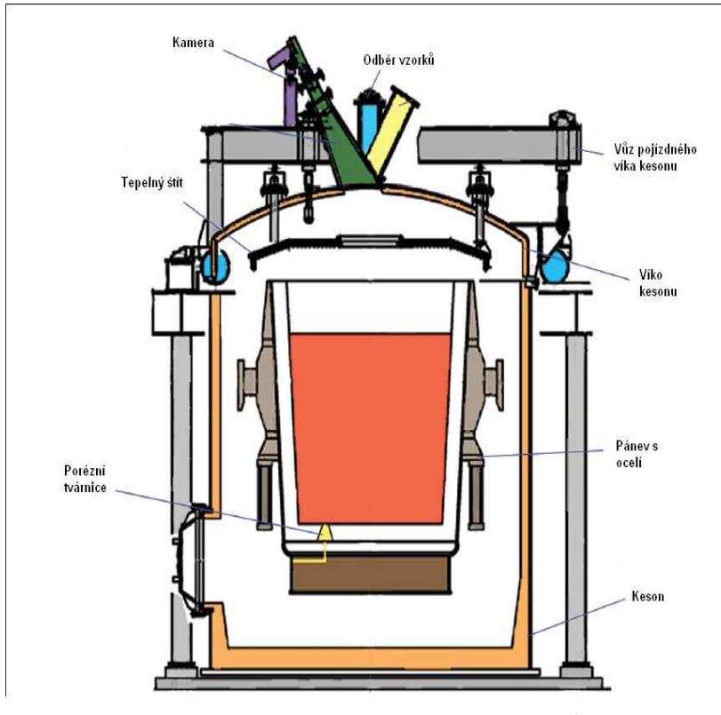
Schema vakuovací stanice
