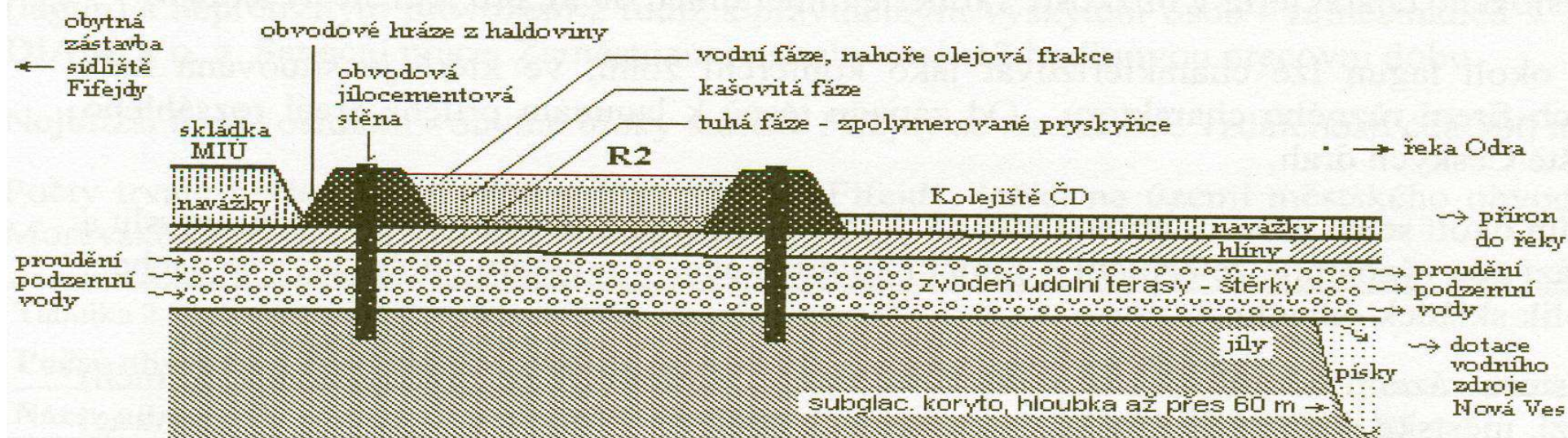
Laguny OSTRAMO - schematický příčný řez
