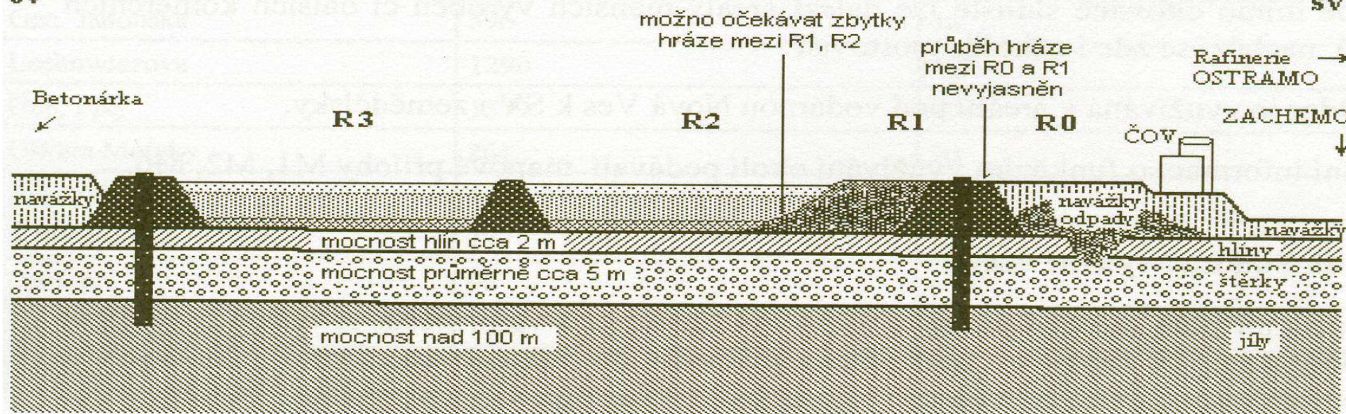
Laguny OSTRAMO - schematický podélný řez
